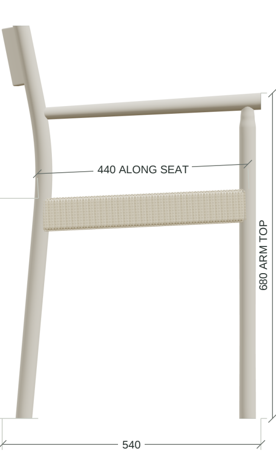
02 SIDE
